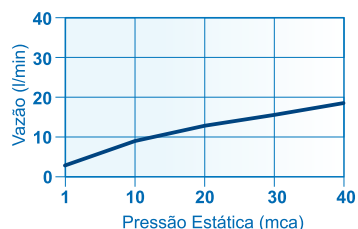
Curva de Vazão x Pressão da Ducha
